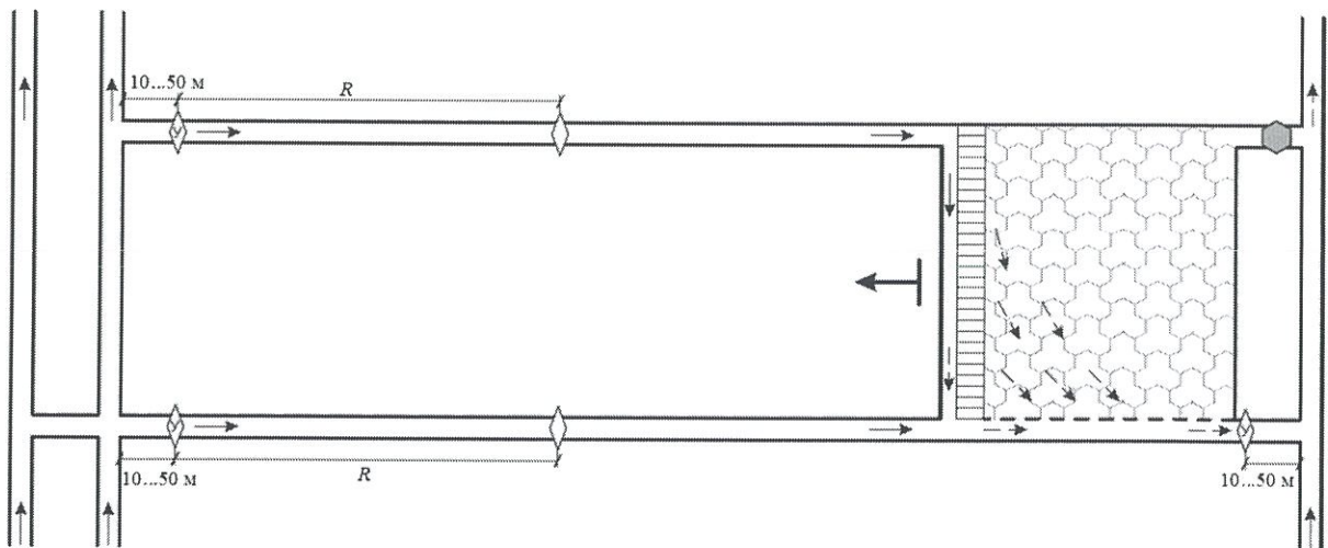
Рисунок 4 – Схема установки средств ВЗГВ для выемочного участка с прямой схемой проветривания
