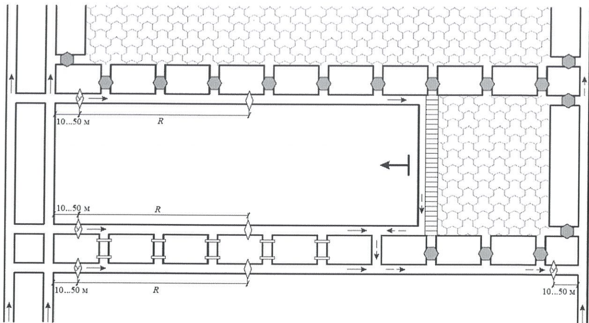
Рисунок 3 – Схема установки средств ВЗГВ для выемочного участка с возвратоточной схемой проветривания, подготовленного спаренными выработками
