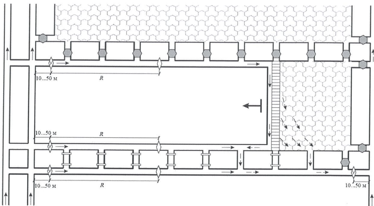
Рисунок 5 – Схема установки средств ВЗГВ для выемочного участка с возвратноточной схемой проветривания и комбинированным направлением выдачи исходящей струи (на заднюю сбойку), подготовленной спаренными выработками
